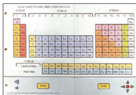
Periodic Table
